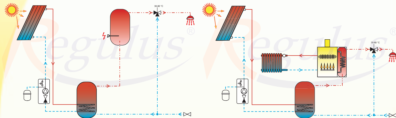
Solární sestava sol 250 KPS11 - přehřev Přehřev pro stávající elektrický zásobník teplé vody. schéma Regulus 1004
