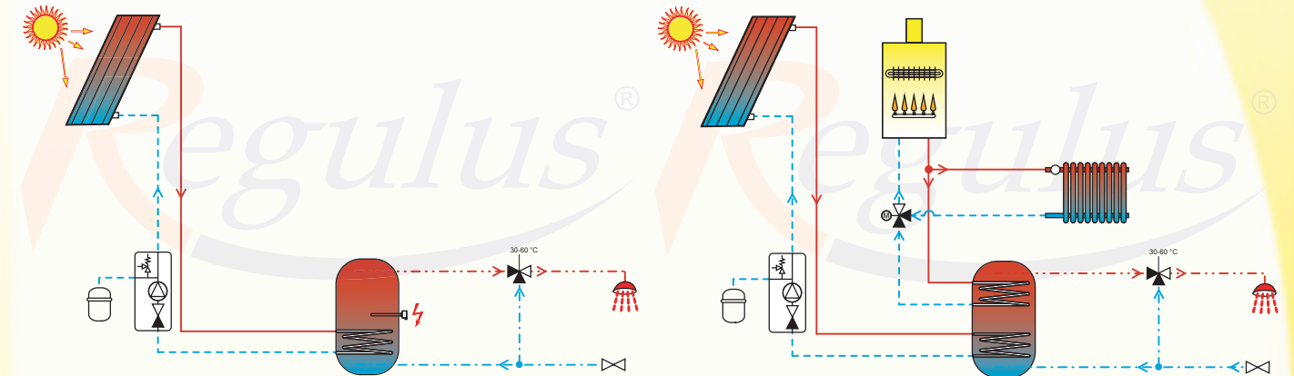
Solární sestava sol 250 KPS11EL - dohřev el. topným tělesem Dohřev elektrickým topným tělesem v solárním zásobníku. schéma Regulus 1001
